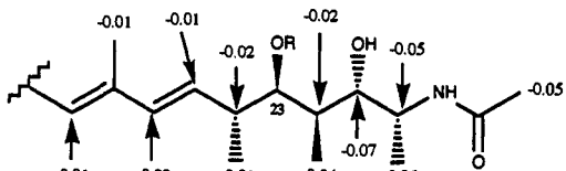
3c R=(+)-( R )-MTPA 3d R=(-)-( S )-MTPA
