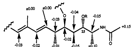
1a R=(+)-( R )-MTPA 1b R=(-)-( S )-MTPA
