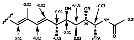
3a R=(+)-( R )-MTPA 3b R=(-)-( S )-MTPA
